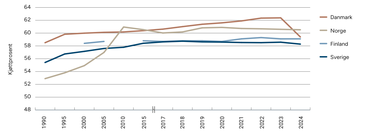
Figur 5.3.f. Kjøttprosentutvikling i Norge, Sverige, Danmark og Finland
